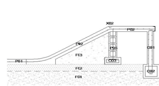
Detalle Rampa
