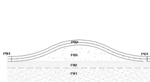
Detalle Duna
